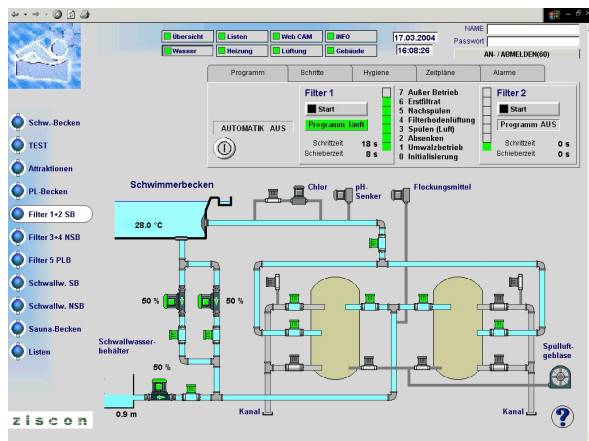
Bild 2: Wassertechnik im Schwimmbad
