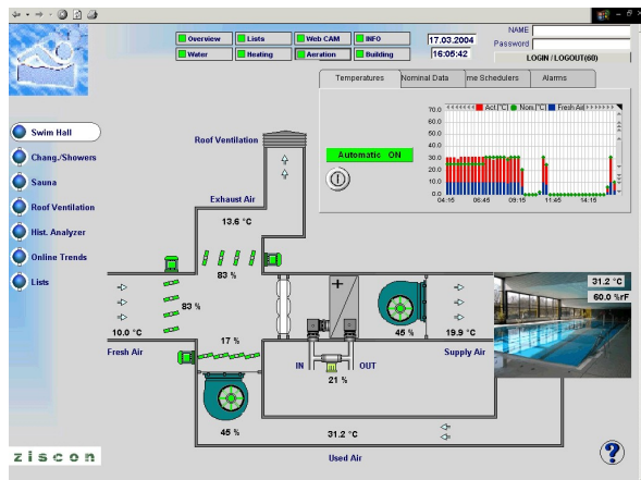
Bild 1: Klimatechnik im Schwimmbad
